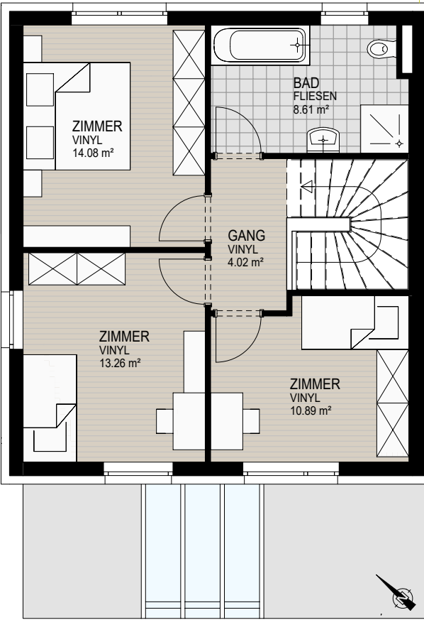
OBERGESCHOSS M 1:100
