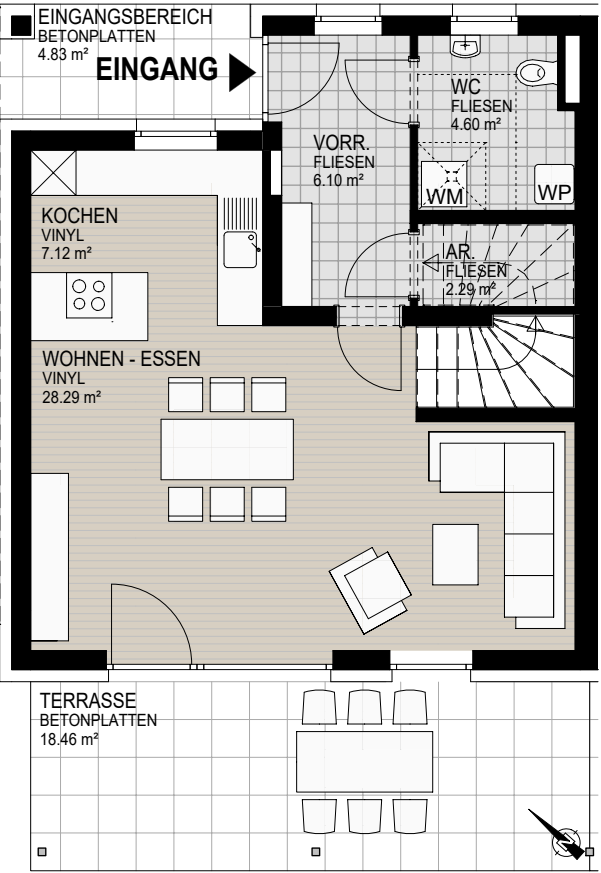
ERDGESCHOSS M 1:100
